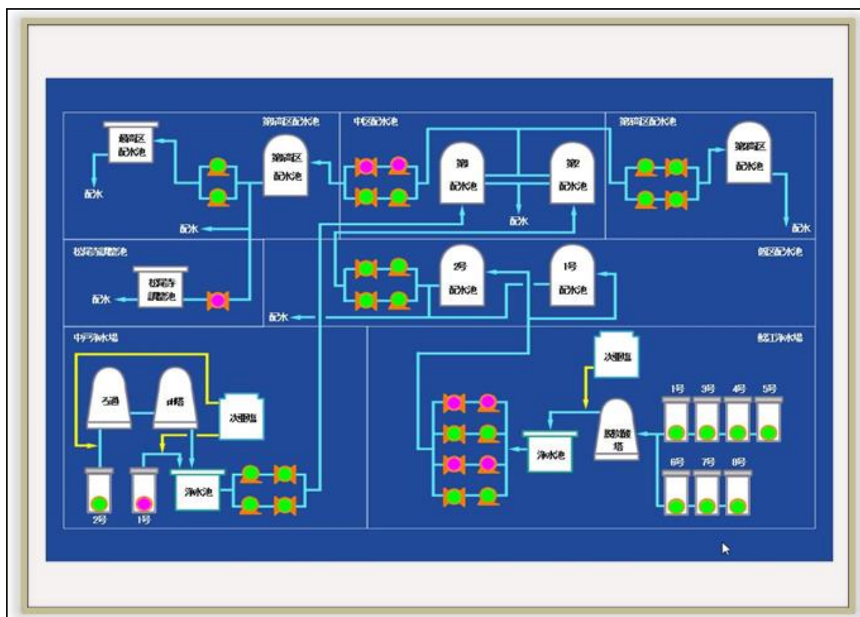
水道施設全体図
