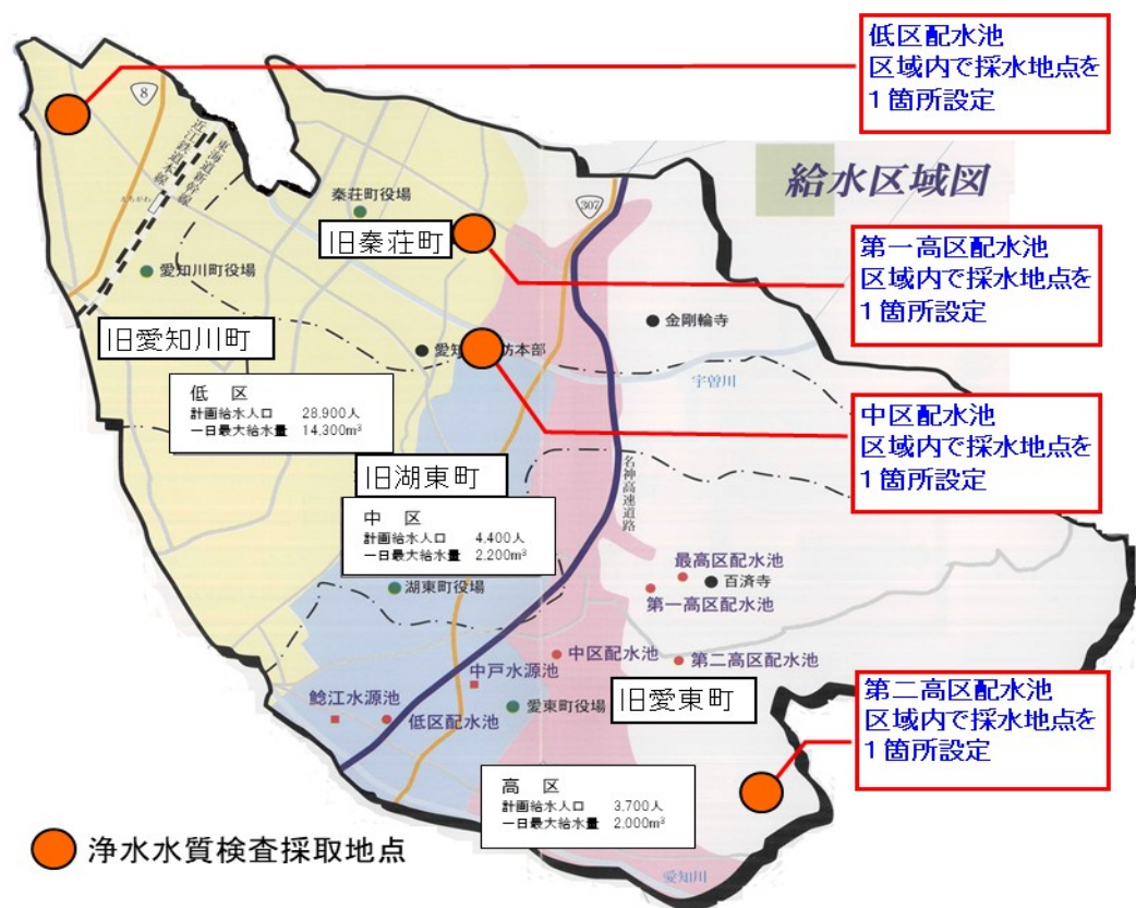
図4-2 給水区域図
